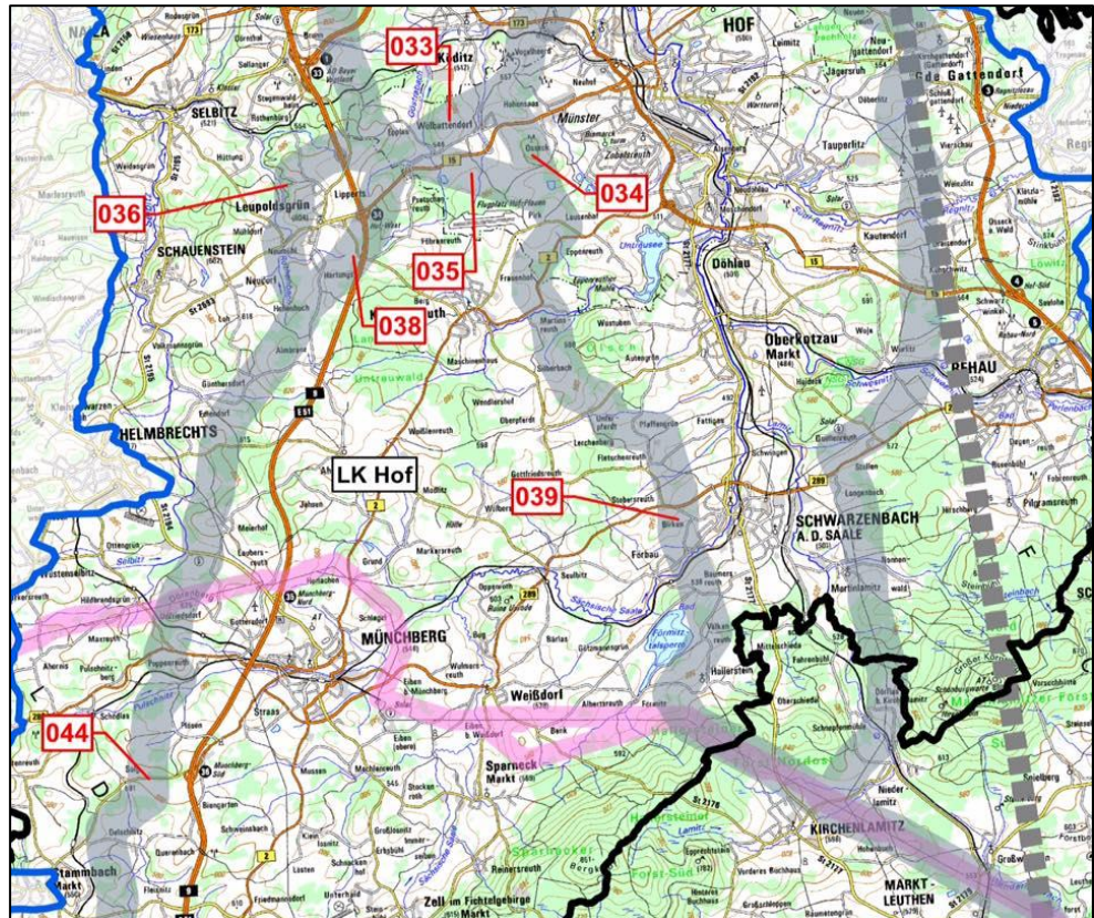
Grau die möglichen Erdkabelkorridore, rosa die möglichen Trassenverläufe des Ostbayernings. Für diesen läuft derzeit noch das Raumordnungsverfahren.
